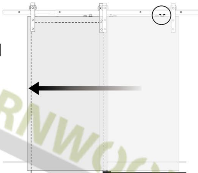
Achteraanzicht softclose systeem in gesloten stand.
