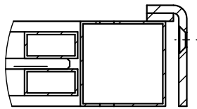
IV 1 : 2
